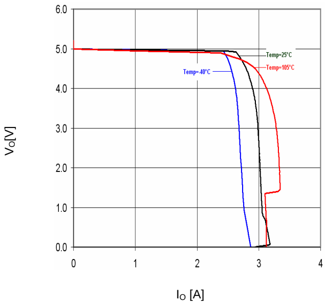
Fig.29 I_o - V_o
