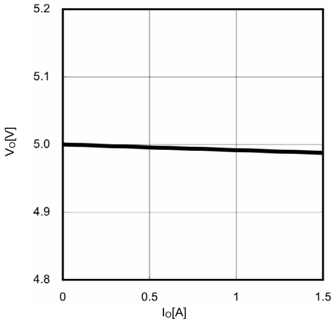
Fig.25 I_O - V_O
