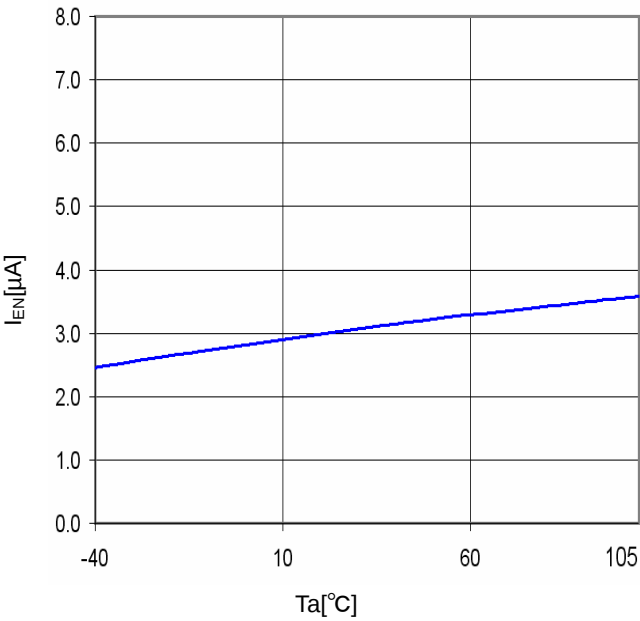
Fig.24 T_a - I_{EN}
