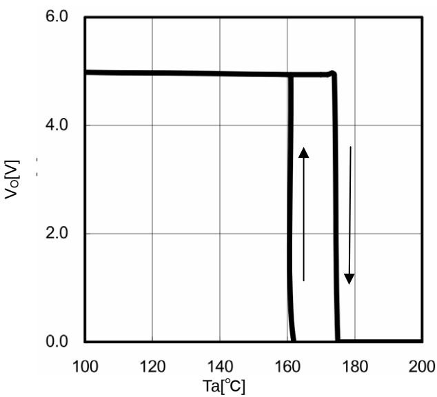
Fig.28 TSD ( I_O=0 mA)
