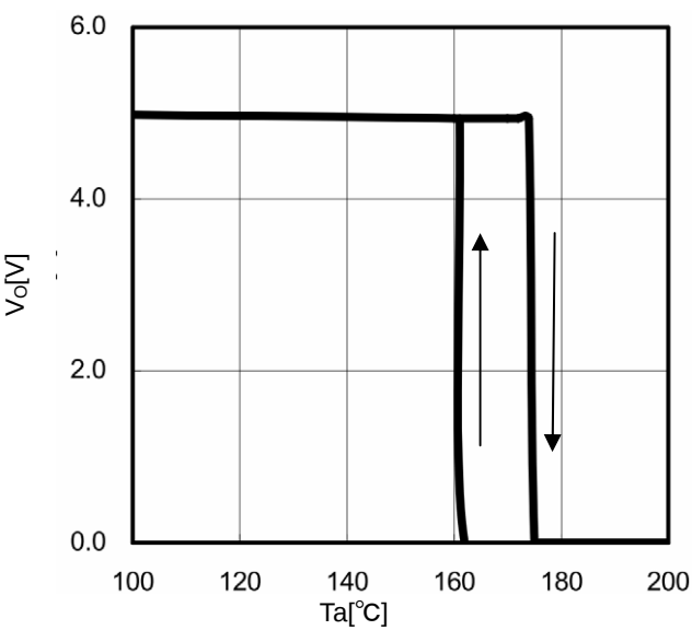
Fig.28 TSD ( I_o=0\text{mA} )
