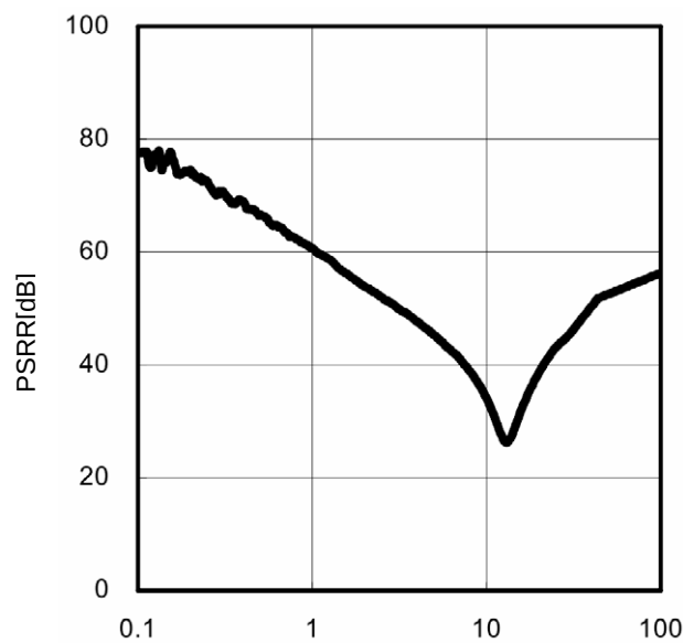
Fig.33 PSRR(I_O=0mA)
