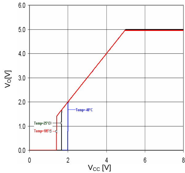
Fig.27 V_{cc}-V_o ( I_o=0\text{mA} )
