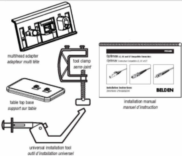
Connector installation tools Outils d'installation du connecteur
