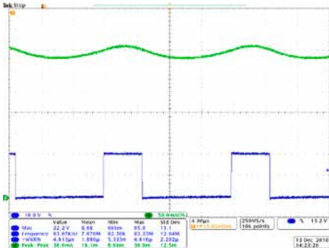
Fig.1: 20V Input
