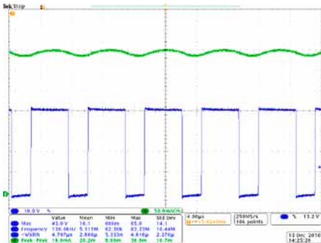
Fig.3: 40V Input
