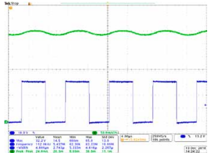
Fig.2: 30V Input
