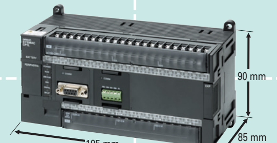
CP1L-M60D
