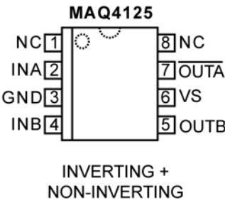
ePad SOIC-8 (ME)
