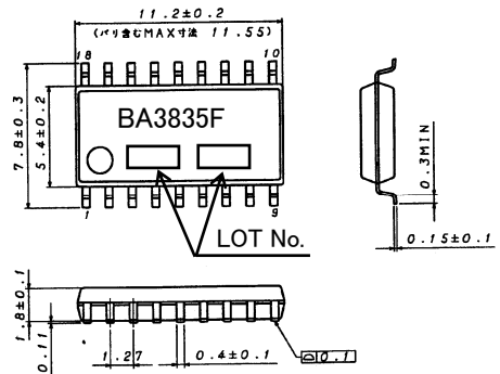
SOP18 (Unit:mm)
