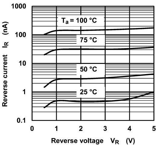
Fig. 9.2 I_R - V_R
