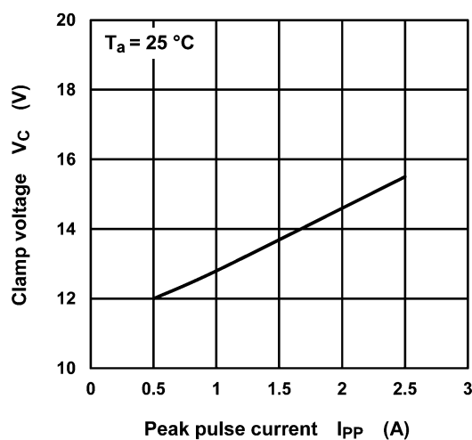
Fig. 6.2.1 V_C - I_{PP}
