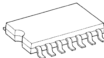
SOP14-P-300-1.27
