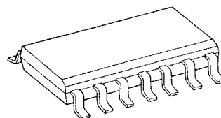
SOL14-P-150-1.27
