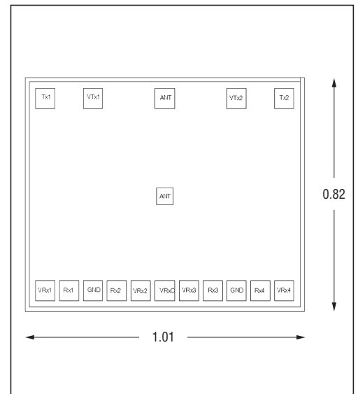
Die Layout
