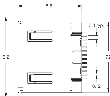
Receptacle
