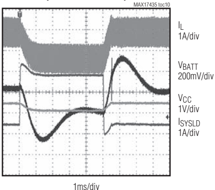
SYSTEM LOAD TRANSIENT (0A \rightarrow 3A \rightarrow 0A)
