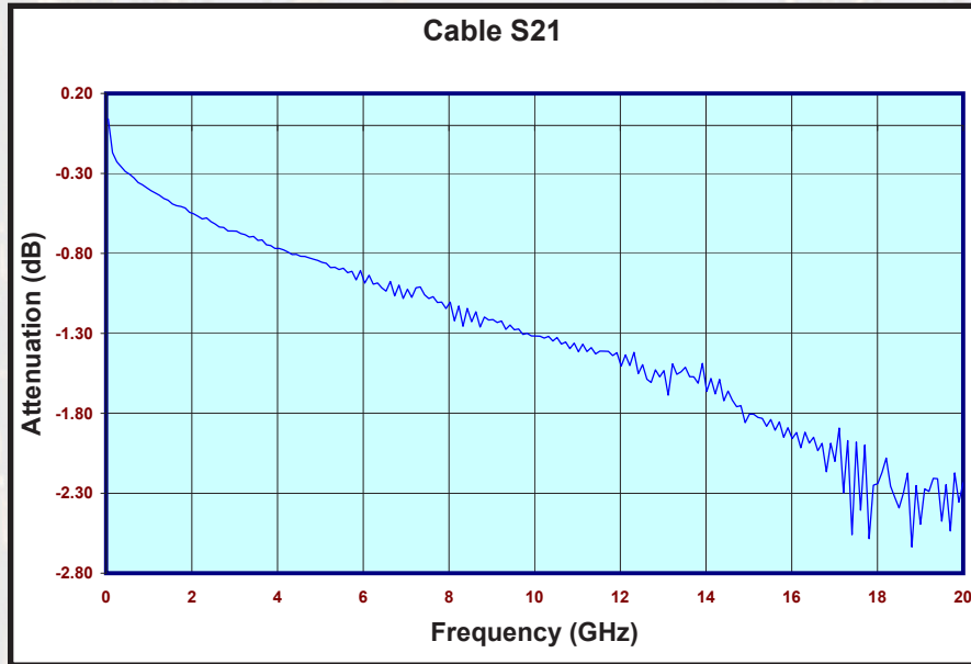
S21 Actual Data Plot PN: CCSMA121-MM-086F-24
