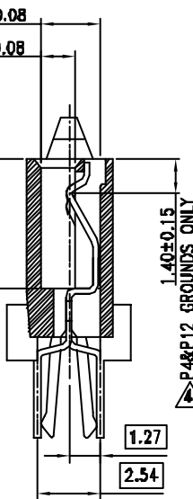
SECTION N-N 2:1
