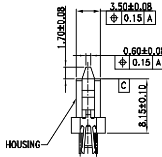
SECTION P-P 2:1
