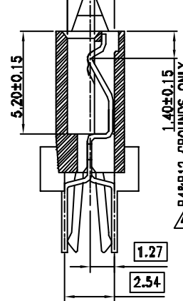
SECTION N-N 2:1
