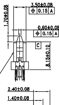
SECTION P-P 2:1
