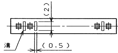
図2 (溝有)
