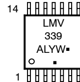
TSSOP-14 CASE 948G
