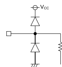
Pin 13 (IS+)
