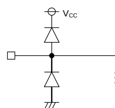
Pin 12 (IS-)
