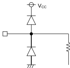
Pin 11 (VOUT)
