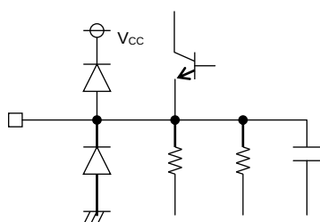
Pin 7 (VREG)
