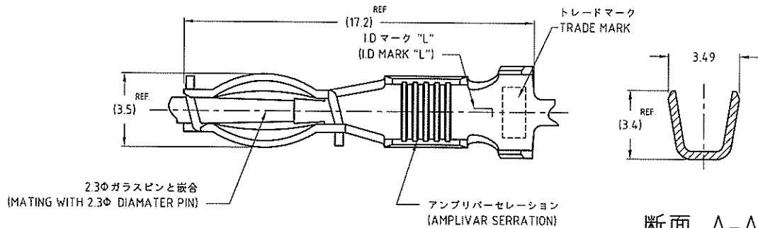
断面 A-A (SECT.)
