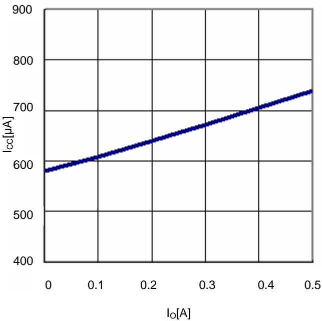
Fig.20 I_o - I_{cc}
