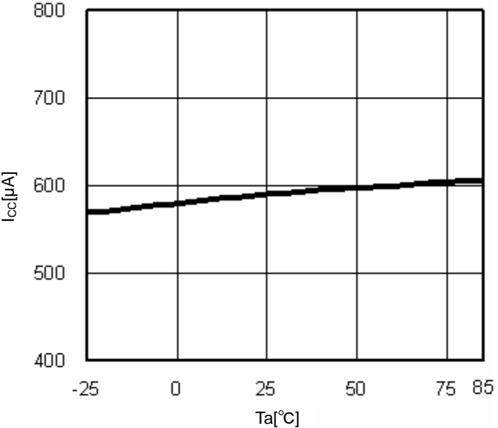
Fig.10 T_a-I_{CC}
