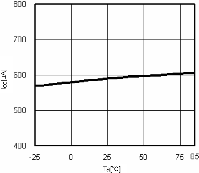
Fig.10 T_a-I_{CC}
