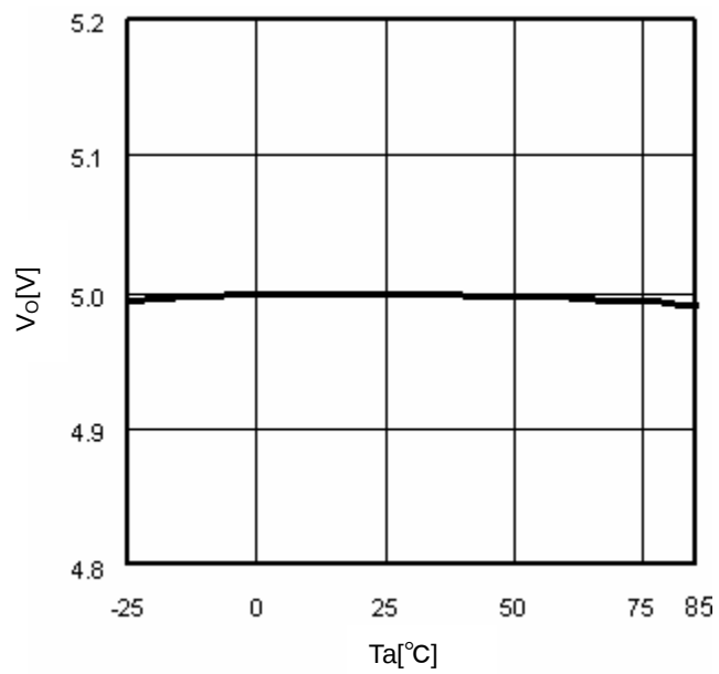
Fig.9 T_a-V_O ( I_o=0mA )
