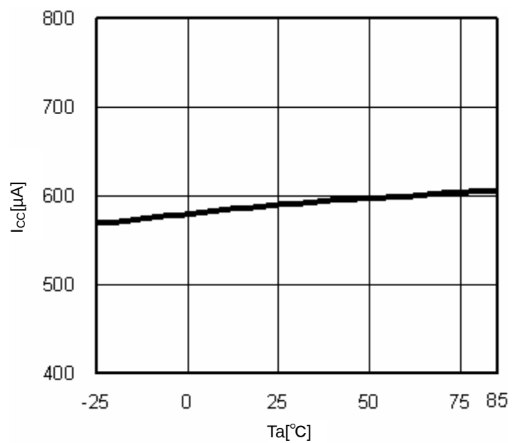
Fig.10 T_a-I_{CC}
