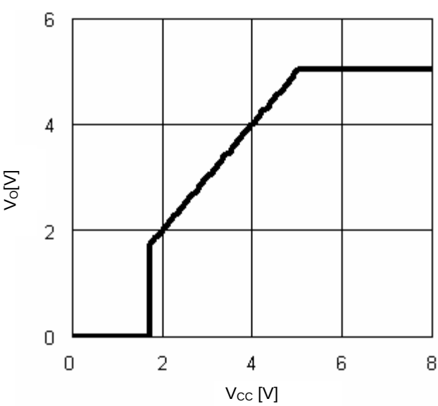
Fig.15 V_{CC}-V_O ( I_O=0mA )
