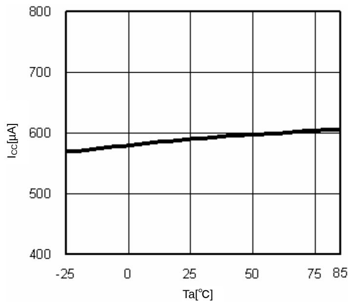
Fig.10 T_a-I_{CC}
