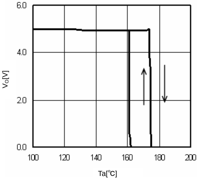
Fig.16 TSD ( I_O=0mA )
