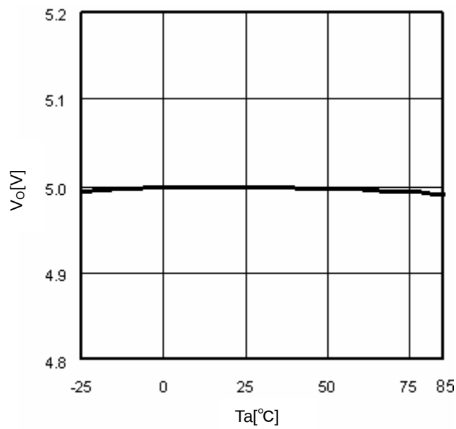
Fig.9 T_a-V_O ( I_o=0mA )
