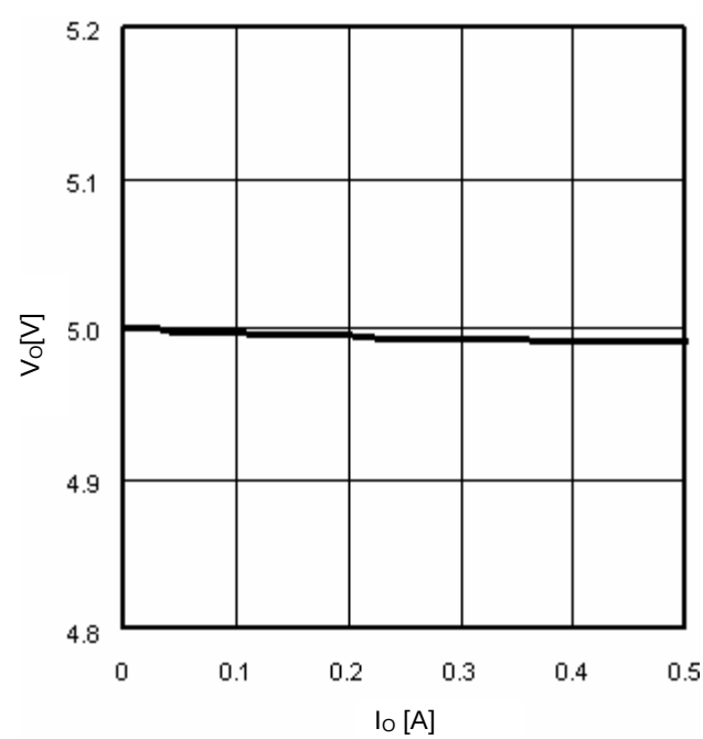
Fig.13 I_O - V_O
