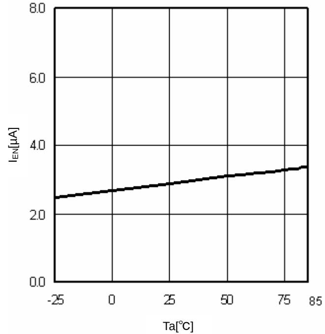
Fig.12 T_a - I_{EN}
