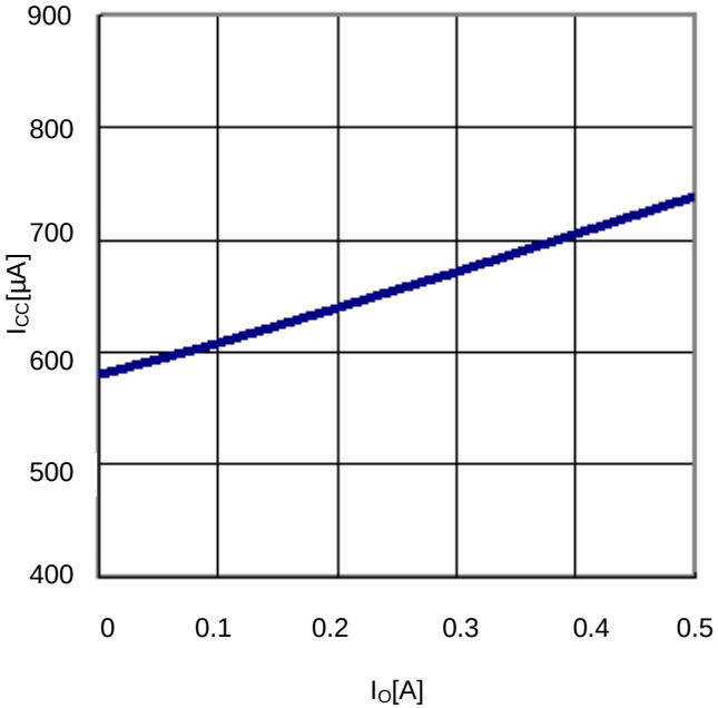
Fig.20 I_o - I_{cc}
