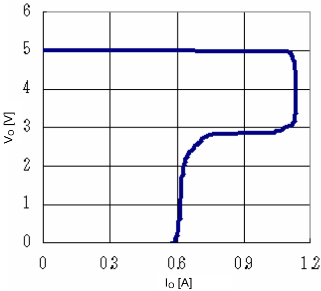
Fig.17 OCP
