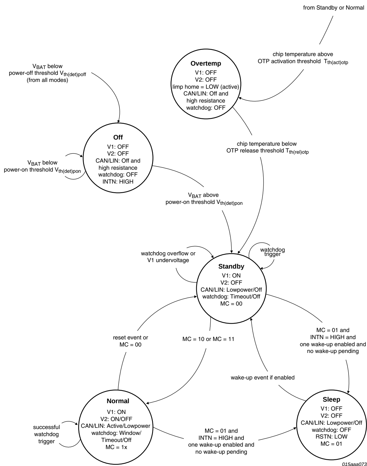
図 3. UJA1078A システムコントローラ
