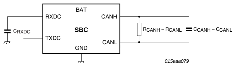
図 17. CAN トランシーバのタイミング試験回路
