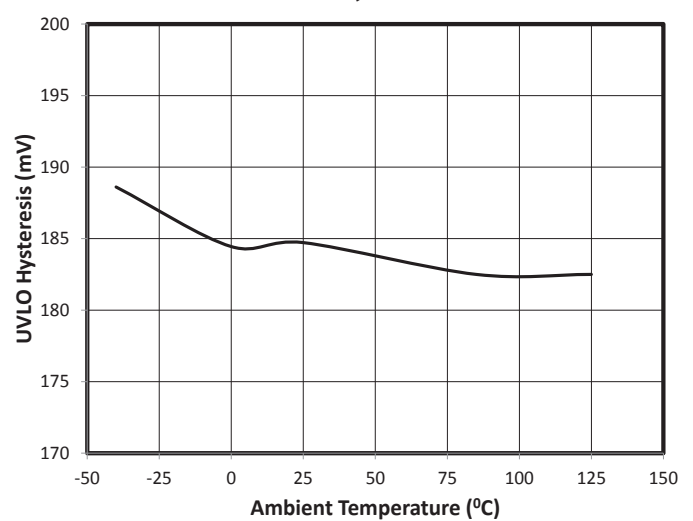
UVLO Hysteresis
