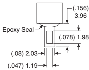
SOLDER LUG
