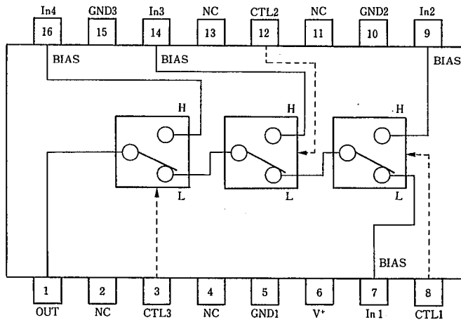
NJM2293D NJM2293M
