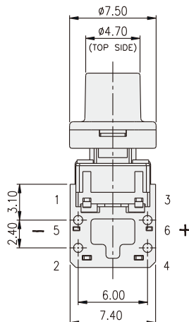
P.C.B. LAYOUT
