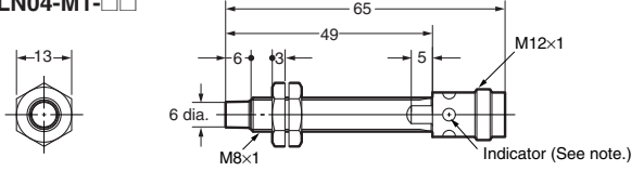
E2A-S08LN04-M1-□□ E2A-M08LN04-M1-□□
