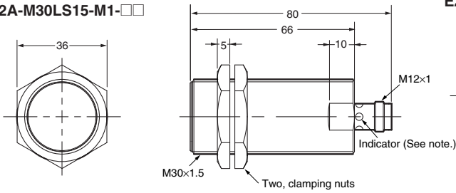
E2A-M30LS15-M1-□□
