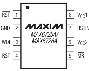
SOT23
