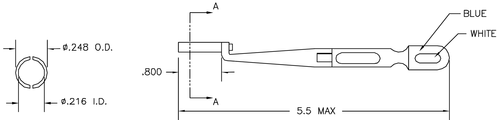
VIEW A-A
