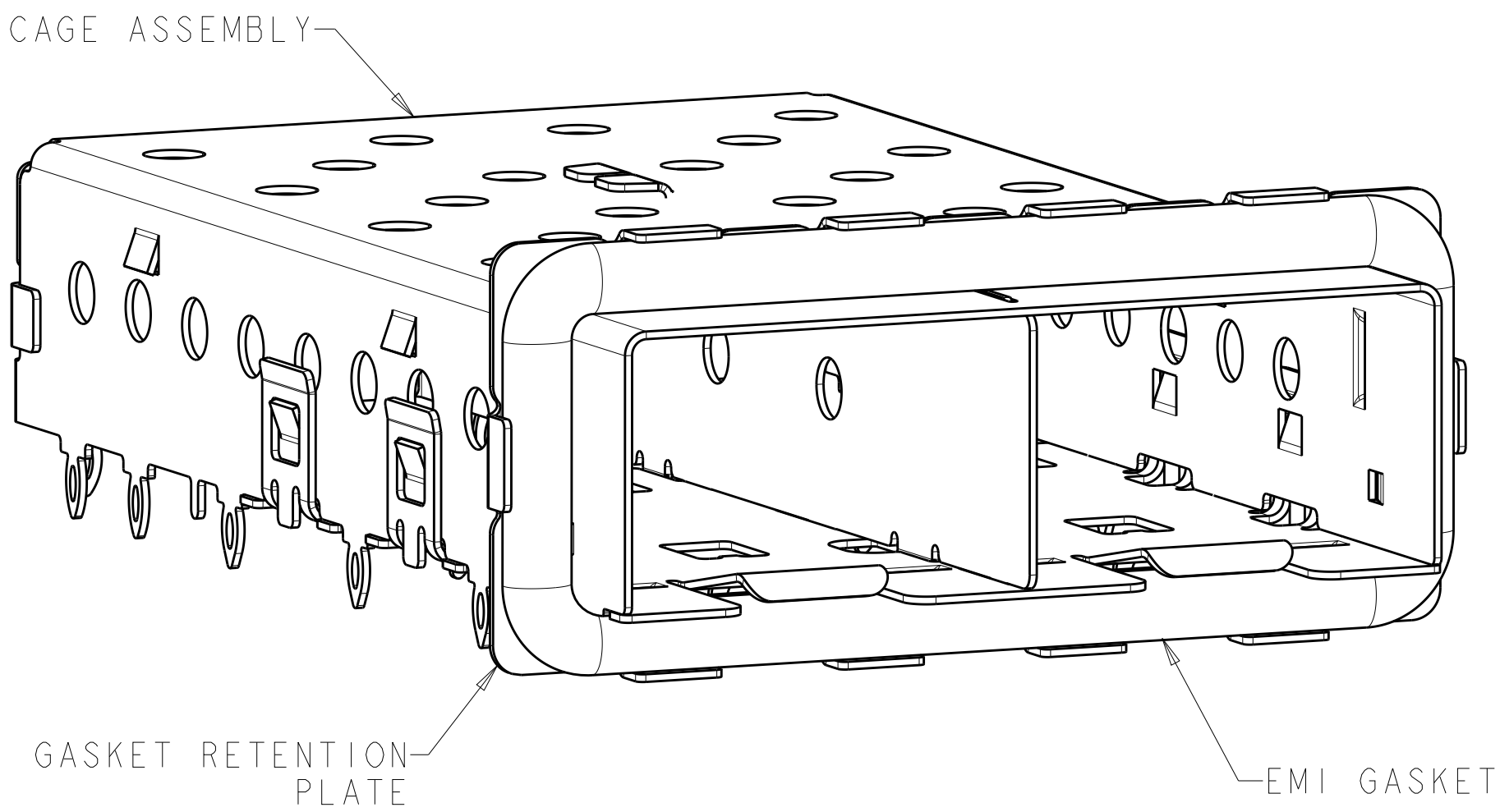
2007181-1 SCALE 5:1
