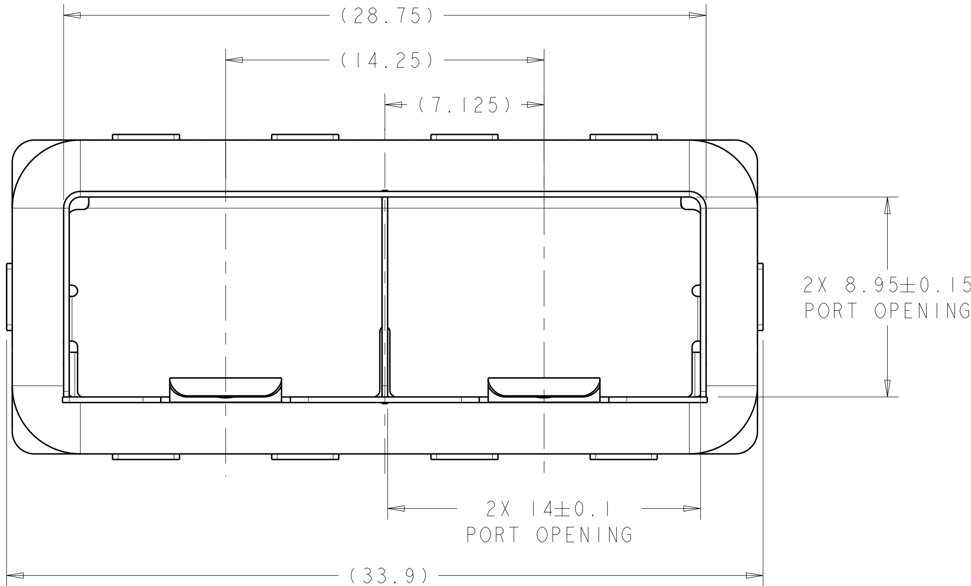
2007181-1 SCALE 5:1
