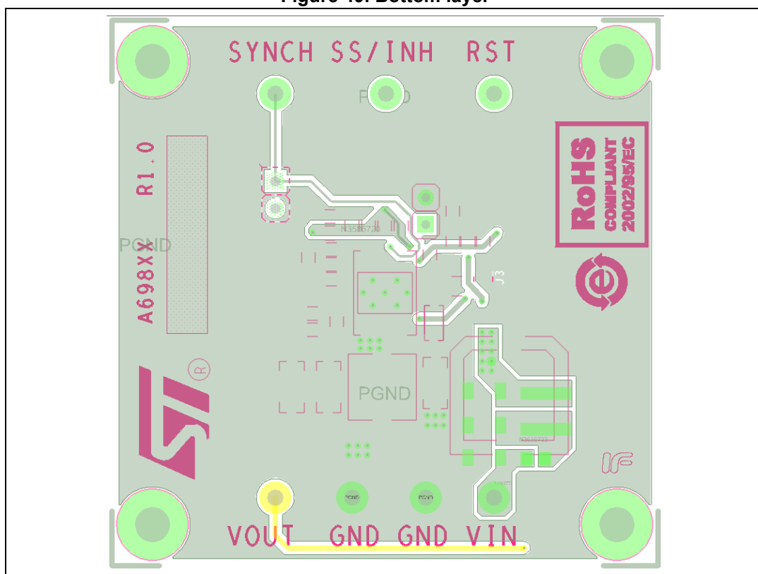
Figure 49. Bottom layer
