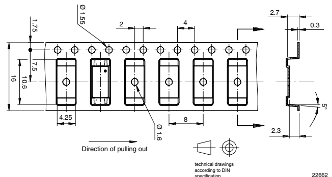
Fig. 21 - Tape Dimensions
