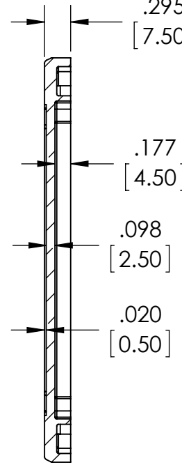
SECTION D-D
