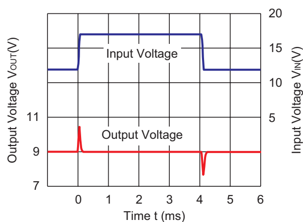
R1514x090B
