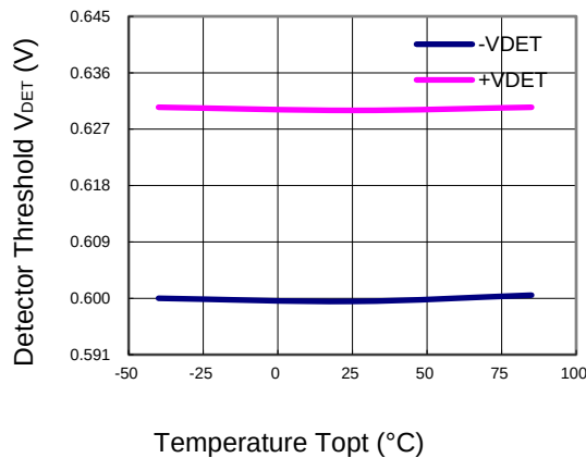
R3118x06xA/C ( V_{DD}=5.3V )
