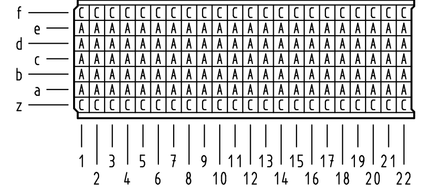
Kontaktbelegung contact loading
