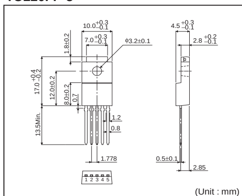
TO220FP-5(V5)
