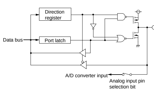
(13) Ports P20-P27
