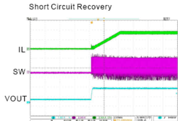
V in =3.3V, V o =1.2V, I o =3.5A
