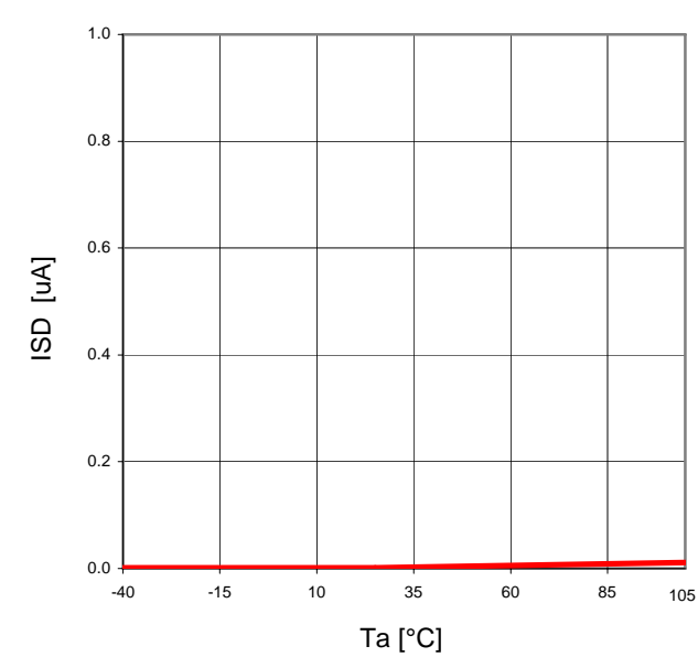
Fig.23 Ta-ISD (VEN=0V)
