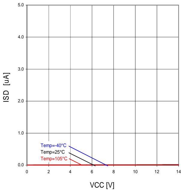
Fig.26 VCC-ISD (VEN=0V)
