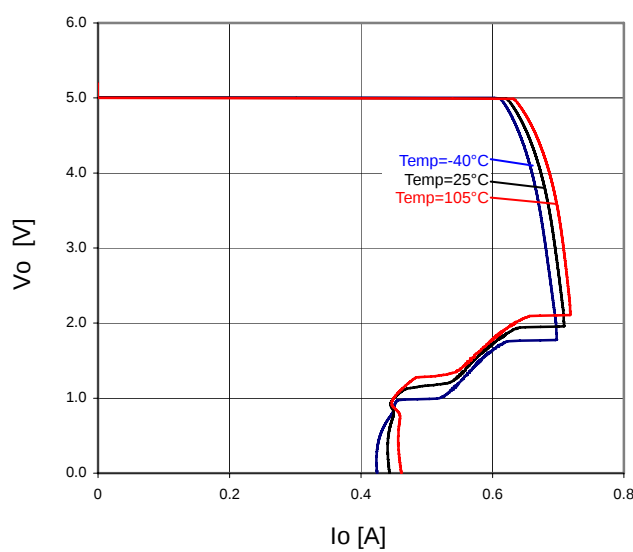
Fig.29 OCP
