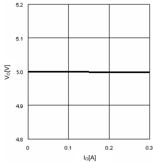
Fig.25 I_O - V_O
