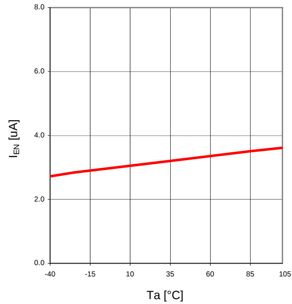
Fig.24 Ta- I_{EN}
