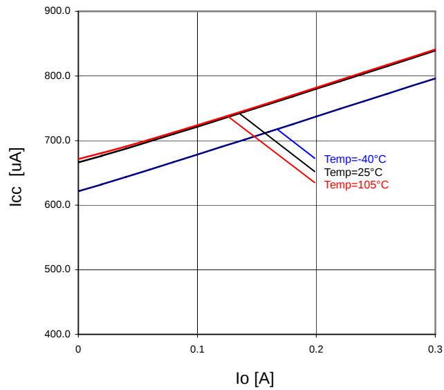
Fig.30 I_o - I_{CC}
