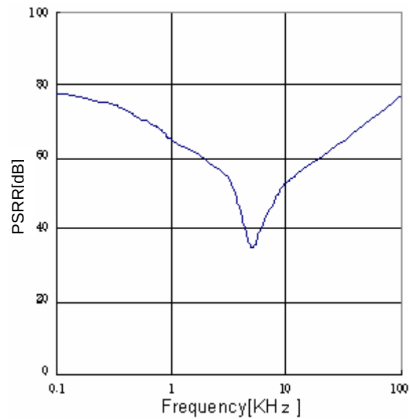
Fig.32 PSRR(Io=0mA)
