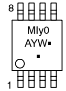
Micro8 MC33164DM CASE 846A
