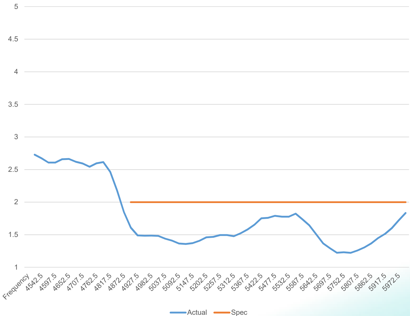
ICEFIN49DMN VSWR
