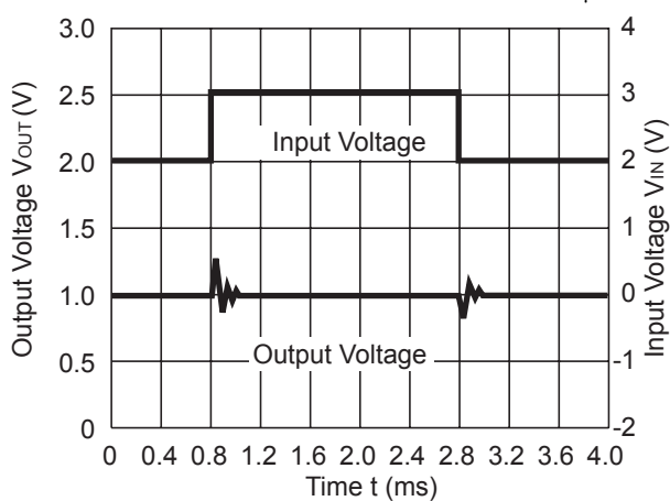
R1161x26xx (ECO=L)
