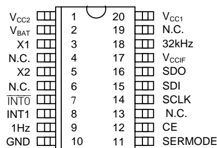
TSSOP (4.4mm)
